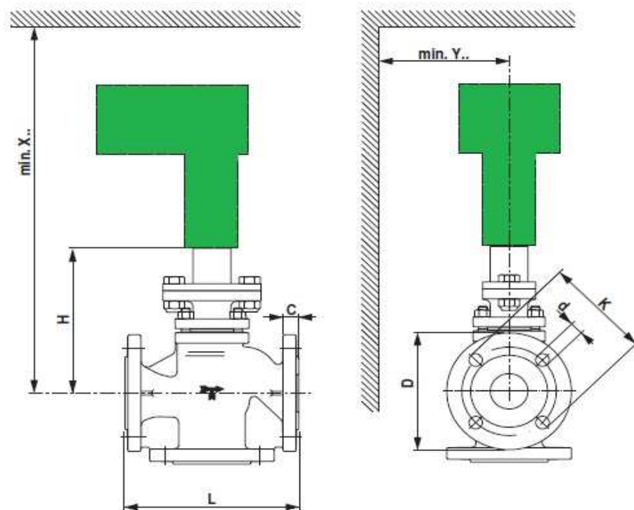
Dimensioni valvole 2-3 vie flangiate PN25
