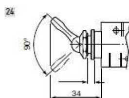
Interruttore - valvole G1/8
