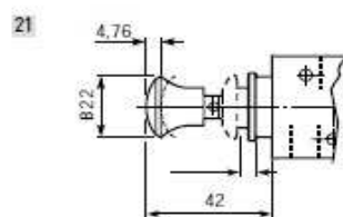
Manopola - valvole G1/8
