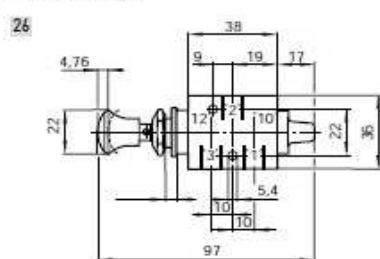
Valvola con manopola di richiamo - valvole G1/8
