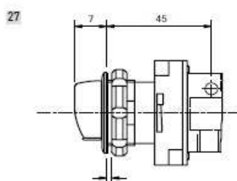
Manopola girevole - valvole G1/8
