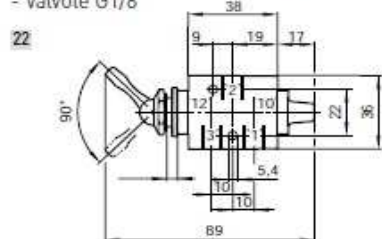
Valvola con molla di richiamo a leva - valvole G1/8
