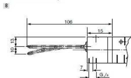
Antenna - valvole G1/8
