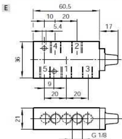
G1/8, 5/2 richiamo a molla, corpo base
