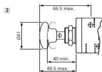
Pulsante - valvole G1/4
