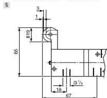
Leva a rulli sensibile - valvole G1/8
