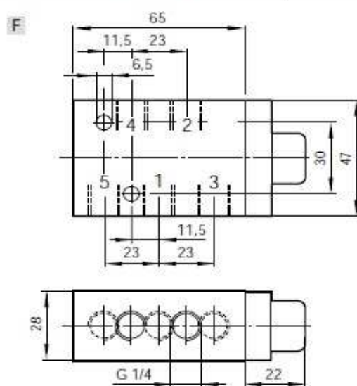
G1/4, 5/2 richiamo a molla, corpo base
