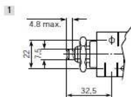
Pulsante - valvole G1/8
