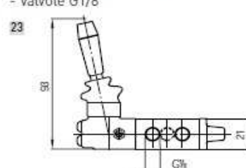
Valvola con molla di richiamo a leva - valvole G1/8
