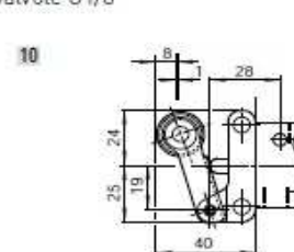
Leva a rulli per lavoro pesante - valvole G1/8
