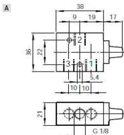
G1/8, 3/2 richiamo a molla, corpo base
