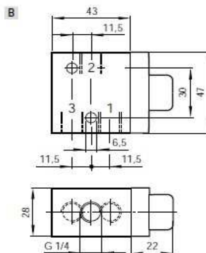
G1/4, 3/2 richiamo a molla, corpo base
