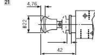
Interruttore leva G1/8" Lever - G1/8"
