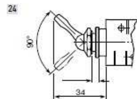
Interruttore leva G1/8" Lever - G1/8"
