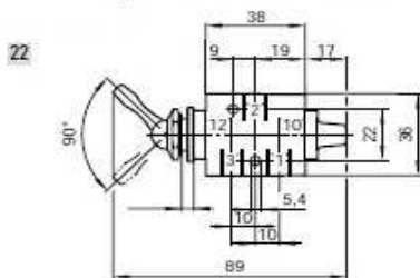
Con molla richiamo leva - G1/8" Lever operated - G1/8"
