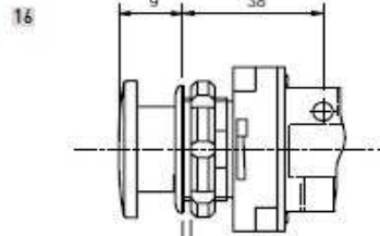
Con molla richiamo leva - G1/8" Lever operated - G1/8"
