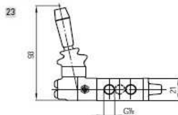
Con molla richiamo leva - G1/8" Lever operated - G1/8"
