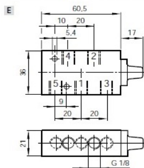
G1/8" - 5/2, ritorno a molla, corpo base G1/8" - 5/2, spring return, basic body
